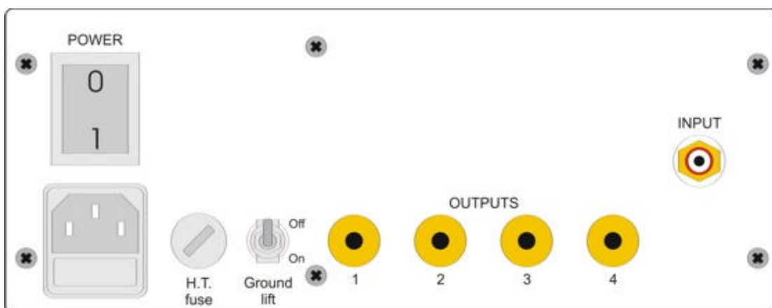
Panel posterior del Amplificador Audion Sterling Mono
