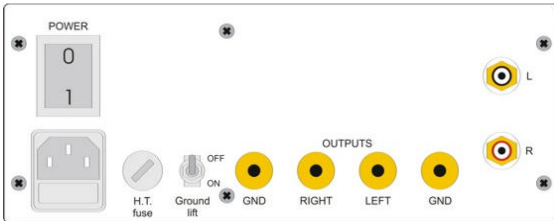
Panel posterior del Amplificador Audion Sterling Stereo
