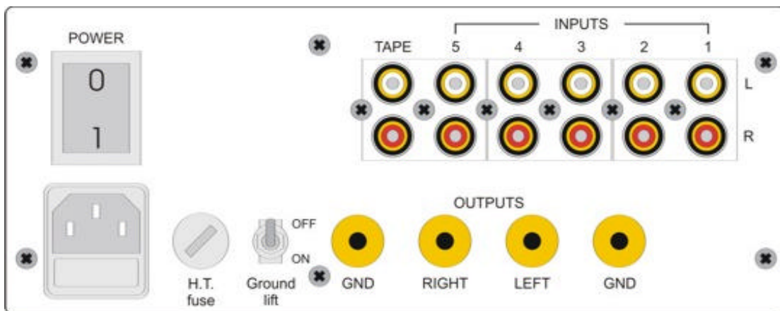
Panel posterior del Amplificador Audion Sterling Integrado / Remoto
