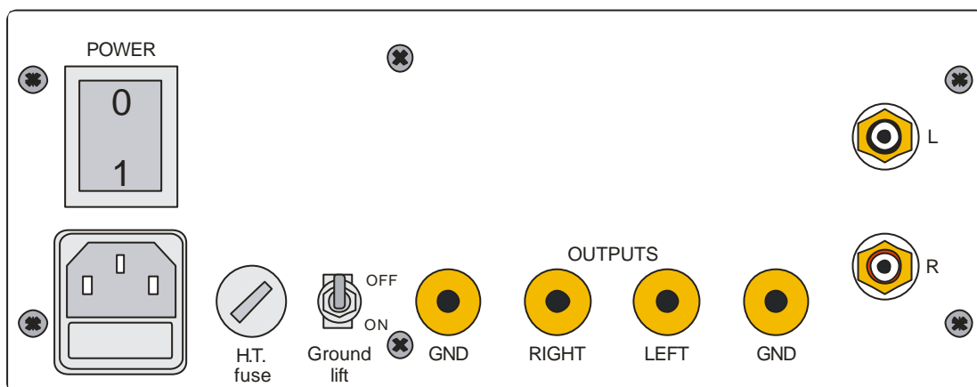
Audion Silver Night Stereo Förstärkare Bakre Panel
