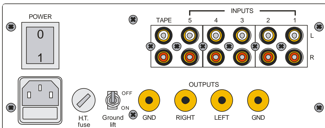
Audion Silver Night Integrerad / Fjärrstyrd Förstärkare Bakre Panel
