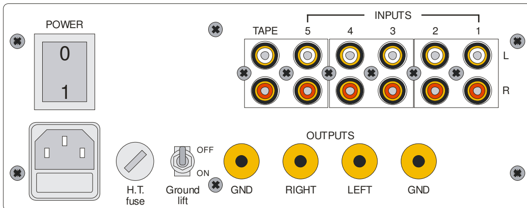
Rückansicht des Audion Silver Night Integrated Verstärkers mit Fernbedienung
