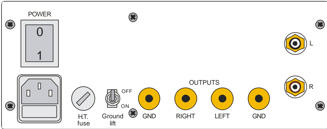
Aménagement de la face arrière de l'amplificateur Audion Silver Night Stereo
