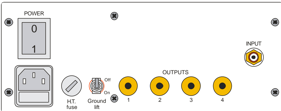
Aménagement de la face arrière de l'amplificateur Audion Silver Night Mono-block
