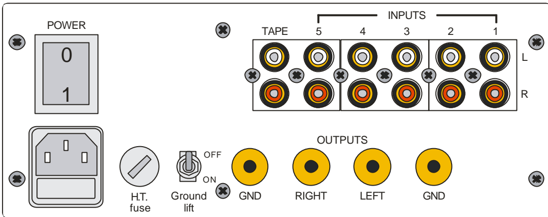
Aménagement de la face arrière des amplificateurs Audion Silver Night Integrated et Remote
