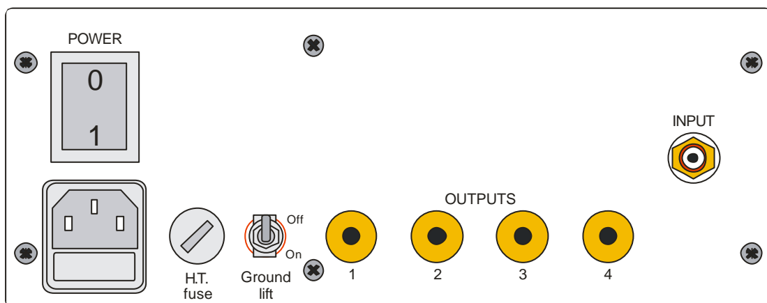
Aménagement de la face arrière des blocs monophoniques Golden Night d’Audion
